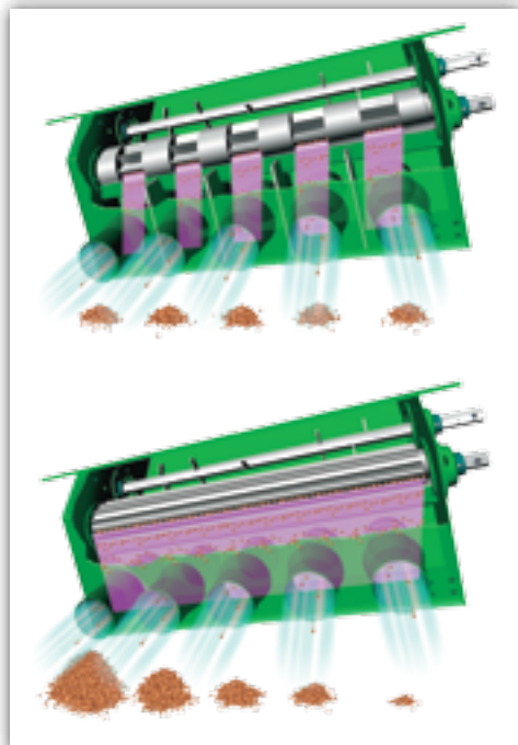
Высевающий аппарат с отдельными отсеками
